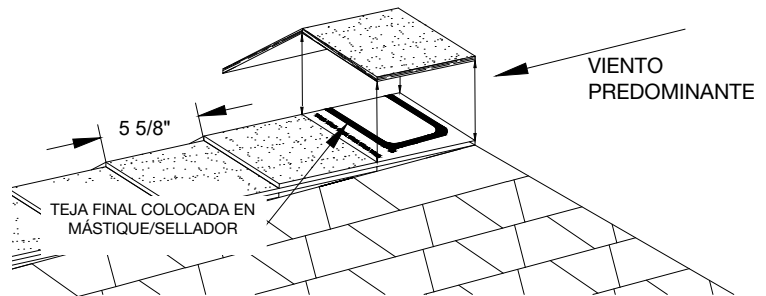
Figura 23 - Instalación de las tejas RidgeFlex®; tapa extrema colocada en mástique (la flecha marca la dirección de los vientos predominantes)
