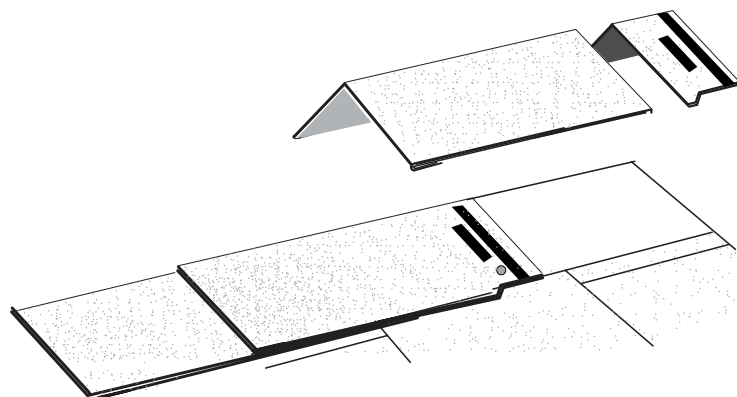
Figura 26 - Teja EZ-Ridge® cortada para crear una tapa extrema
