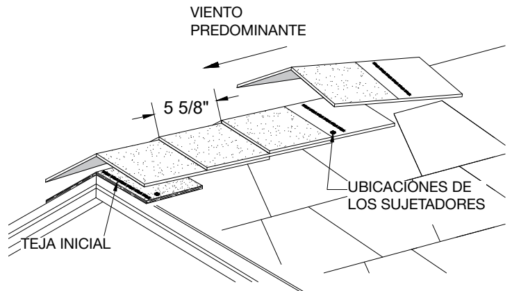
Figura 22 - Emplazamiento y sujeción de las tejas RidgeFlex®, manteniendo la exposición de 5⅝"
