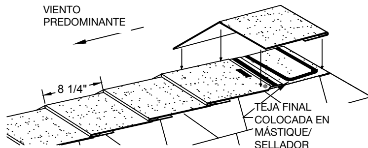
Figura 27 - Posicionamiento y sujeción opcional de la tapa extrema EZ-Ridge®
