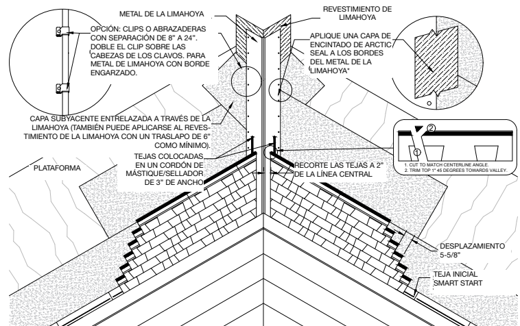
Figura 12 - Aplicación en limahoya metálica abierta
