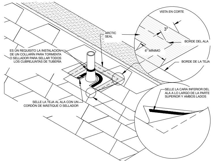
Figura 14 - Aplicación de cubrejuntas de tubería de ventilación
