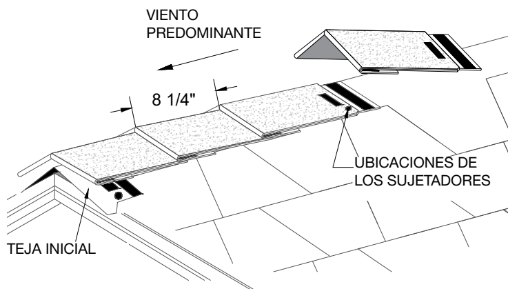
Figura 25 - Emplazamiento y sujeción de las tejas EZ-Ridge®, manteniendo la exposición de 8\frac{1}{4} "
