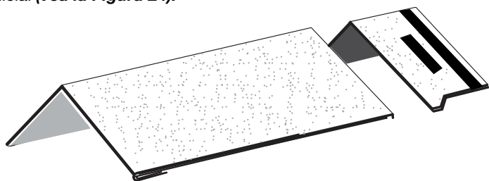
Figura 24 - Corte de una teja EZ-Ridge® para hacer una teja inicial para limatesas y cumbreras
