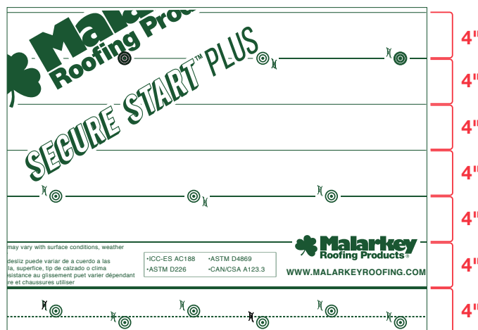
Figura 1 - SecureStart™ Plus tiene líneas de guía de traslapeo de hilada cada 4" (102 mm)
